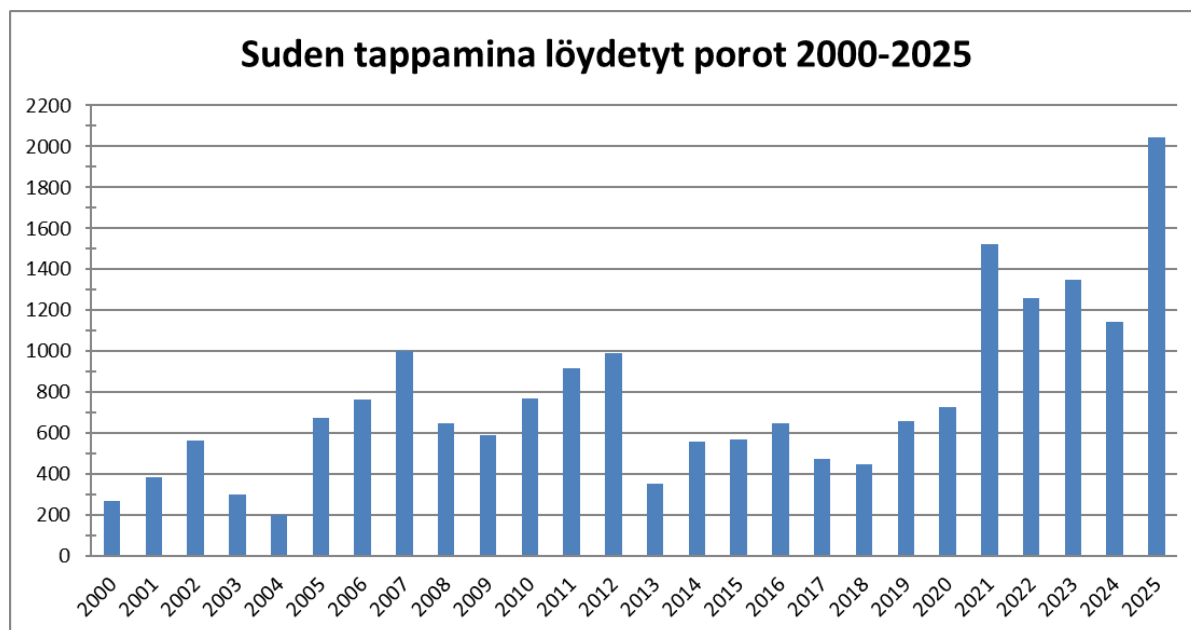
Kuva 1. Suden tappamina löydetyt porot 2000–11.12.2025.
